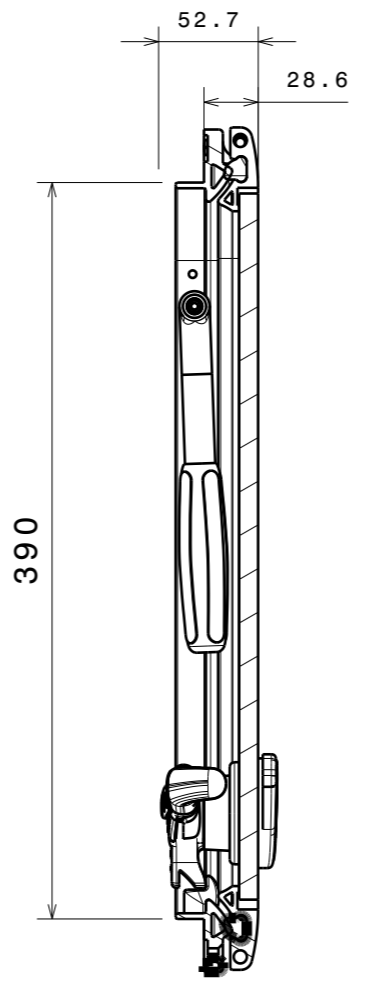
Section A-A Scale: 1:4
